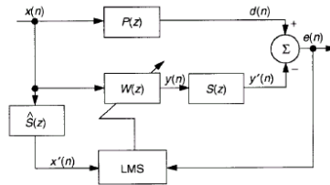
Gambar Diagram blok sistem ANC menggunakan algoritma FXLMS
