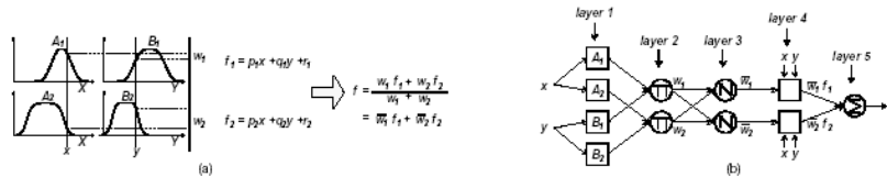
Gambar (a) Model fuzi Sugeno orde-satu dua maukan dengan dua aturan (b) Kesamaan arsitektur ANFIS-nya.
