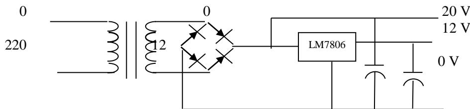
Gambar Rangkaian Catu Daya
