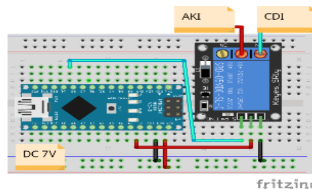
Gambar 8. Perancangan Modul Relay untuk CDI
