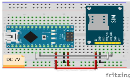
Gambar 5. Perancangan Modul Sim800L
