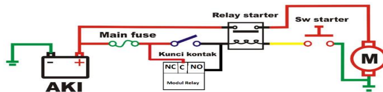
Gambar 7. Perancangan Aliran Listrik Kunci Kontak
