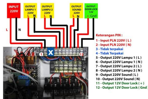
Gambar 2. Rangkaian ASB
