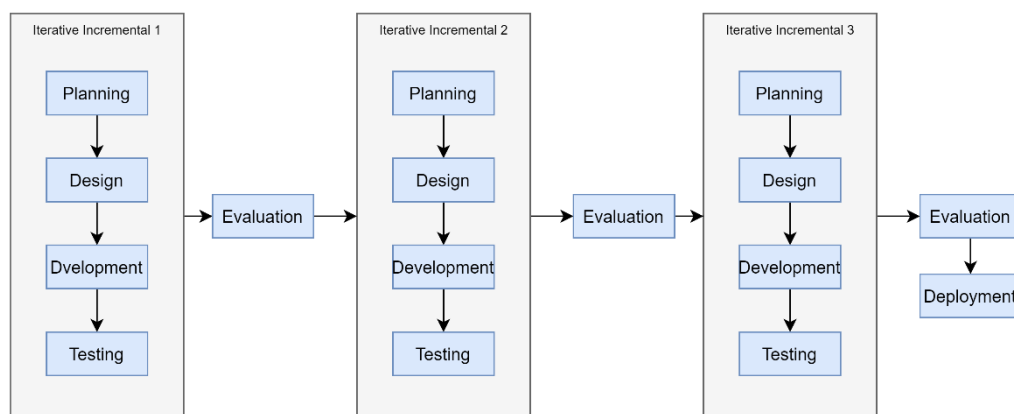
Gambar 1. Tahapan pada metode pengembangan Iterative Incremental
