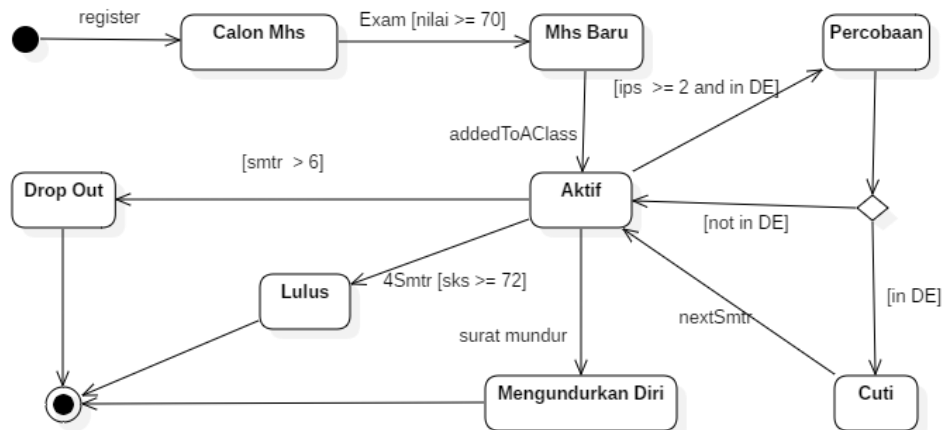
Gambar 7. State Diagram Status Mahasiswa
