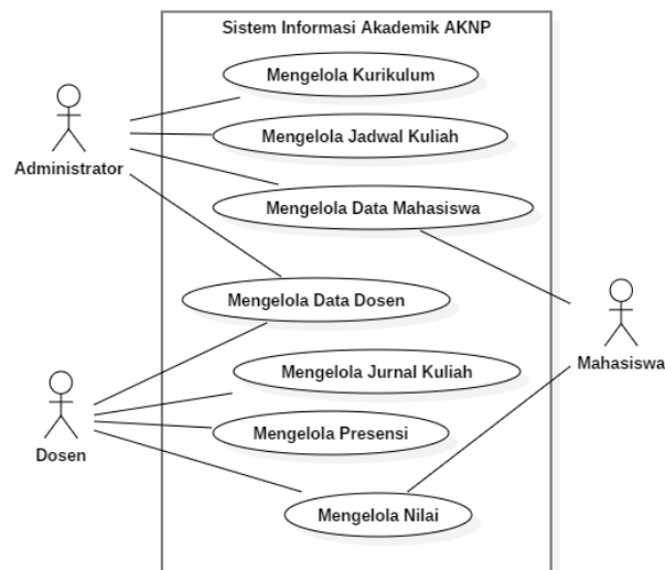
Gambar 4. Use Case Diagram Sistem Informasi Akademik AKNP
