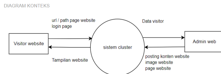
Gambar 3. Diagram Konteks
