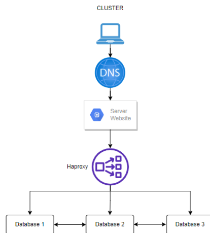
Gambar 2. Desain Sistem
