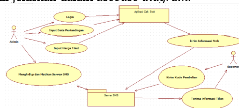
Gambar 3. Perancangan Use Case Diagram
